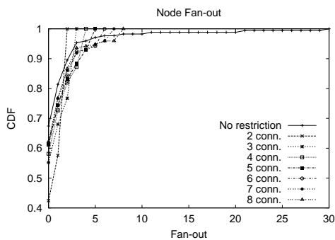
Fig. 17. Fan-out distribution.
