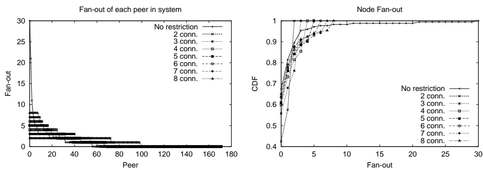
Fig. 14. Fan-out distribution.
