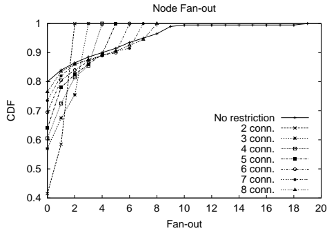
Fig. 11. Fan-out distribution.
