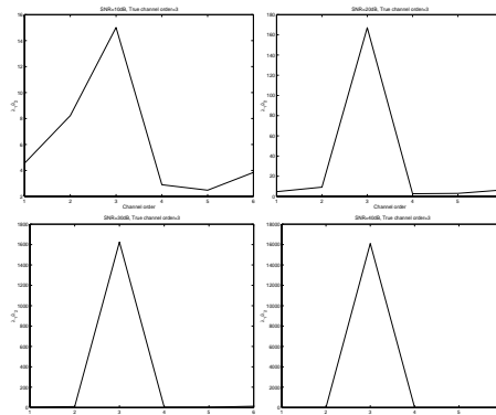
FIG. 3: Détection de l'ordre du canal.
