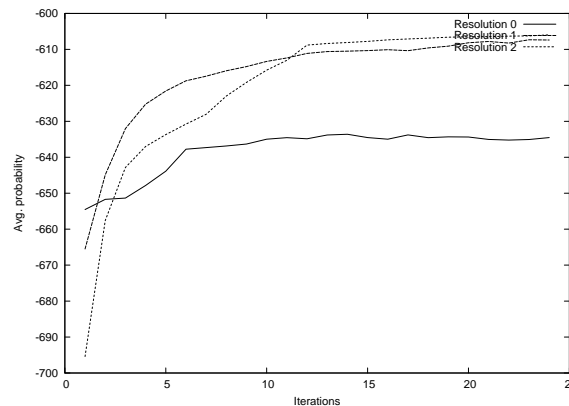
Figure 12. Probabilité totale Durant l'entraînement.
