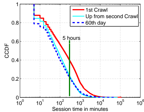
Figure B.6: La CCDF des longueurs de sessions pour différents ensembles de pairs.
